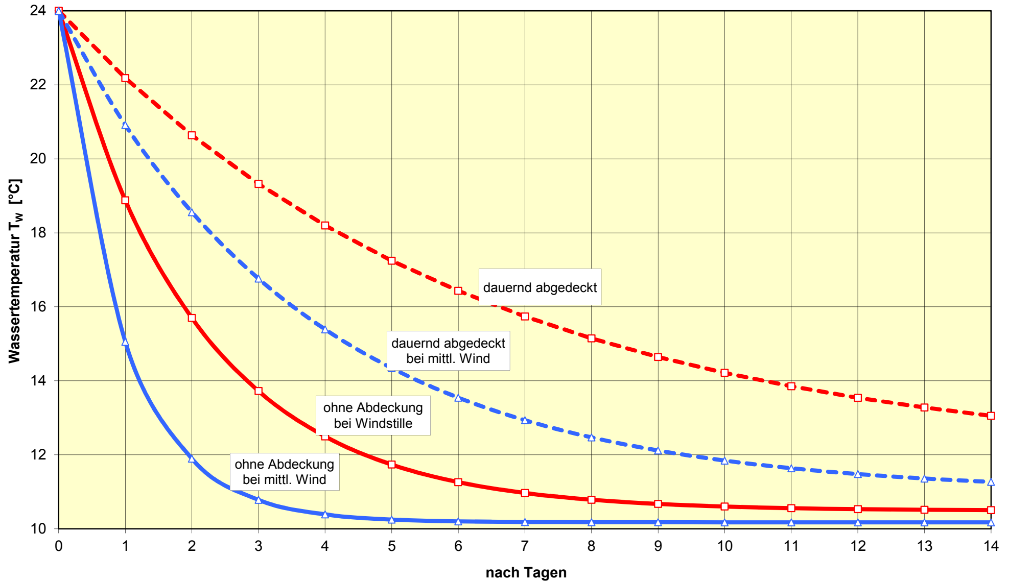
Bild 4: Wasserabkühlung bei Schlechtwetter ohne Heizung ohne / mit Abdeckung beginnend bei T_w = 24^\circ\text{C} , T_L = 10^\circ\text{C}
